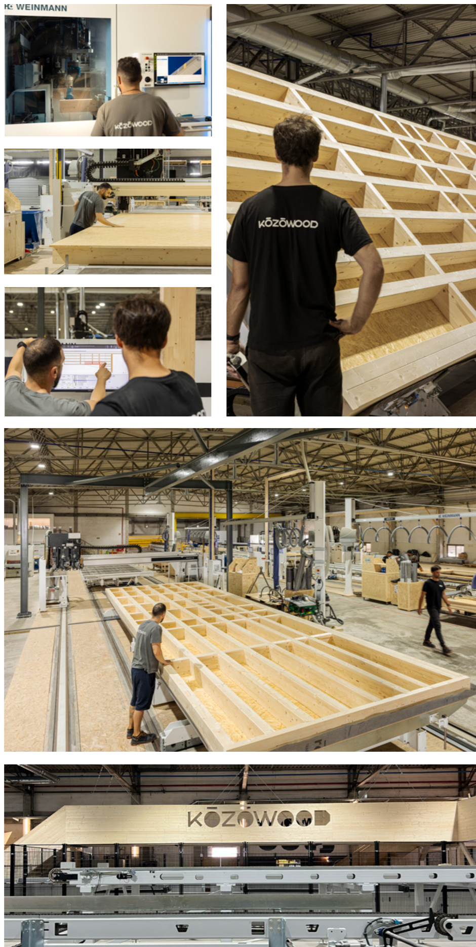
Photos : Utilisation d'une installation pour la taille de charpentes, de tables de montage et de ponts multifonctions dans l'usine de Kōzōwood.
