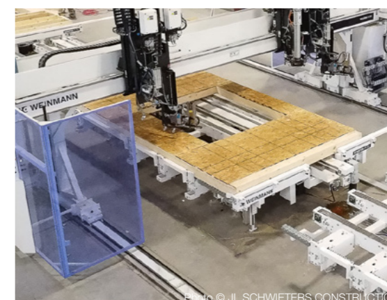
Photos : Création et usinage automatisés des éléments à l'aide des FRAMETEQ et WALLTEQ.
